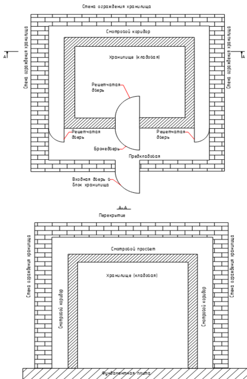
Рисунок 1 – Схематичное устройство хранилища ценностей
